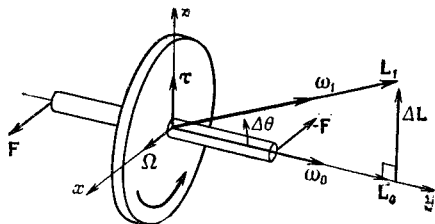
Фиг. 20.2. Гироскоп.
