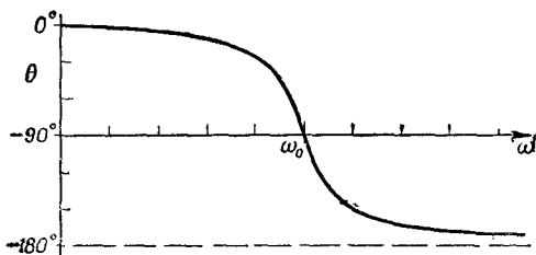
Ф и г. 23.3. График зависимости \theta от \omega .
