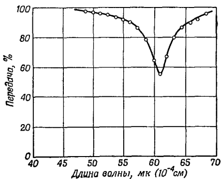
Ф и г. 23.7. Прохождение инфракрасного излучения через тонкую ( 0,17\text{ мк} ) пленку поваренной соли.
