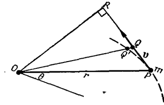
Ф и г. 18.3. Движение частицы относительно оси вращения O .
