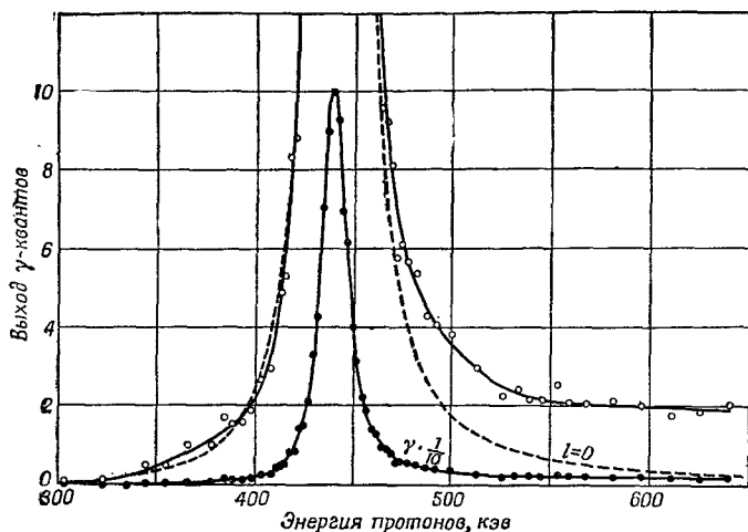
Фиг. 23.9. Зависимость интенсивности \gamma -излучения лития от энергии налетающих протонов.
