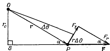
Фиг. 18.2. Вращающий момент, создаваемый силой.
