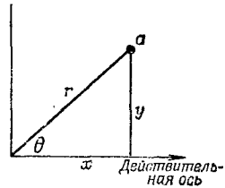
Ф и г. 23.1. Комплексное число, изображенное точкой на «комплексной плоскости».
