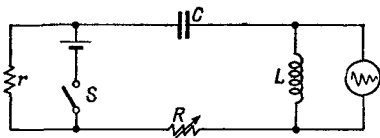
Ф и г. 24.2. Электрическая цепь для демонстраций переходных колебаний.
