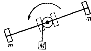
Ф и г. 18.4. Зависимость «инерции вращения» от плеча масс.
