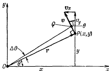
Фиг. 18.1. Кинематика двумерного вращения.
