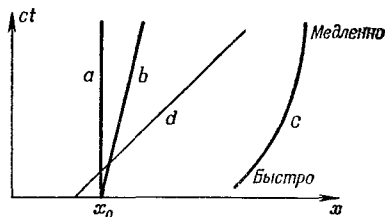
Фиг. 17.1. Пути трех частиц в пространстве-времени.
