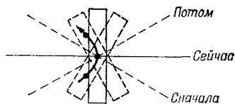
Ф и г. 20.4. Движение частицы вращающегося колеса, показанного на фиг. 20.2. При повороте оси эти частицы движутся по кривой линии.
