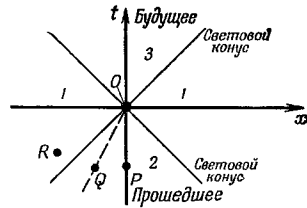
Ф и г. 17.3. Область пространства-времени, окружающая начало координат.
