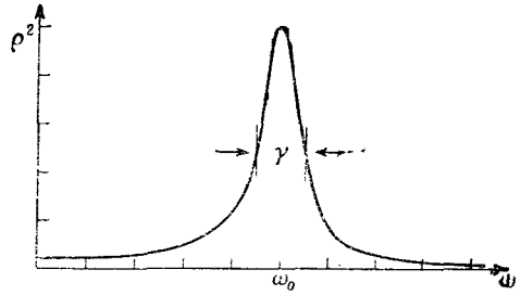
Ф и в. 23.2. График зависимости \rho^2 от \omega .
