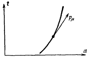
Ф и г. 17.4. Четырехвектор импульса частицы.
