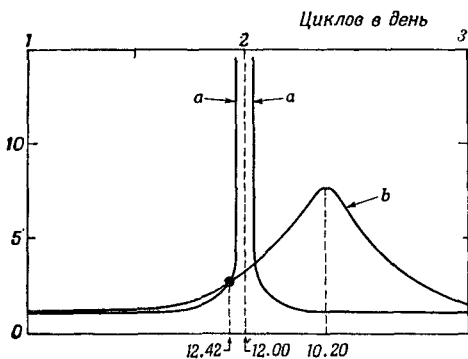
Ф и г. 23.6. Влияние внешнего возбуждения на атмосферу.
