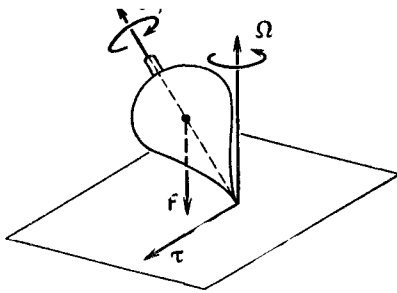
Ф и г. 20.3. Быстро вращающийся волчок.
