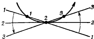
Ф и г. 19.4. Три последовательных положения движущейся по радиусу точки вращающегося стола.
