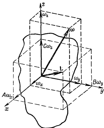
Ф и г. 20.7. Угловая скорость и момент количества движения твердого тела ( A > B > C ).
